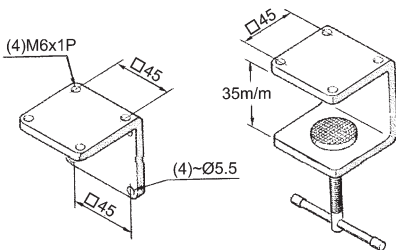
J-L01 AÇI PLAKASI
