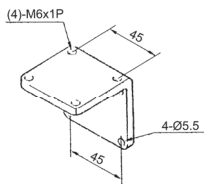
J-L01 AÇI PLAKASI
